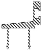
DS 02 Door stop 35mm Door stop in 100 Series
